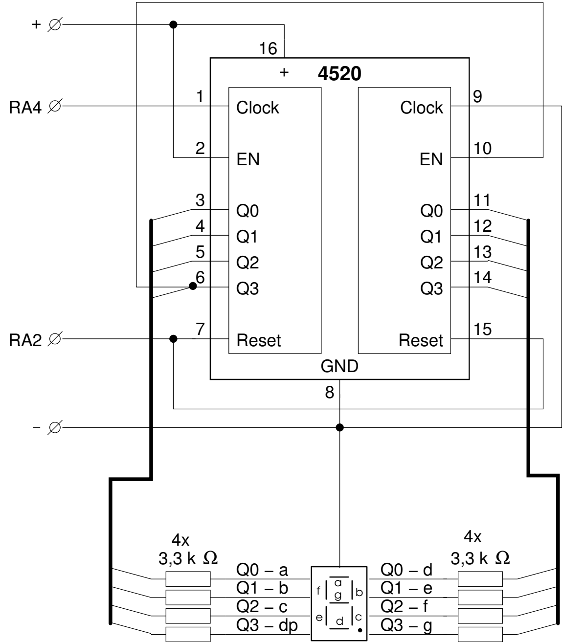
LED Anzeige gemeinsame Kathode
